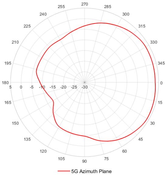
Radio1 Antenna Patterns
